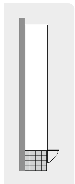
Gemetselde plint met voorgebouwde zitbank
